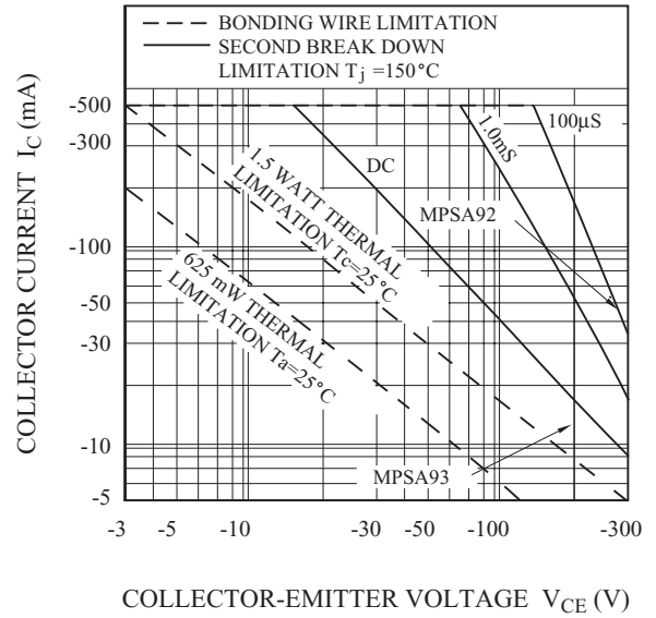
I_C - V_{CE}
