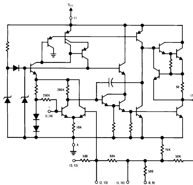
TL/H/7842-1
